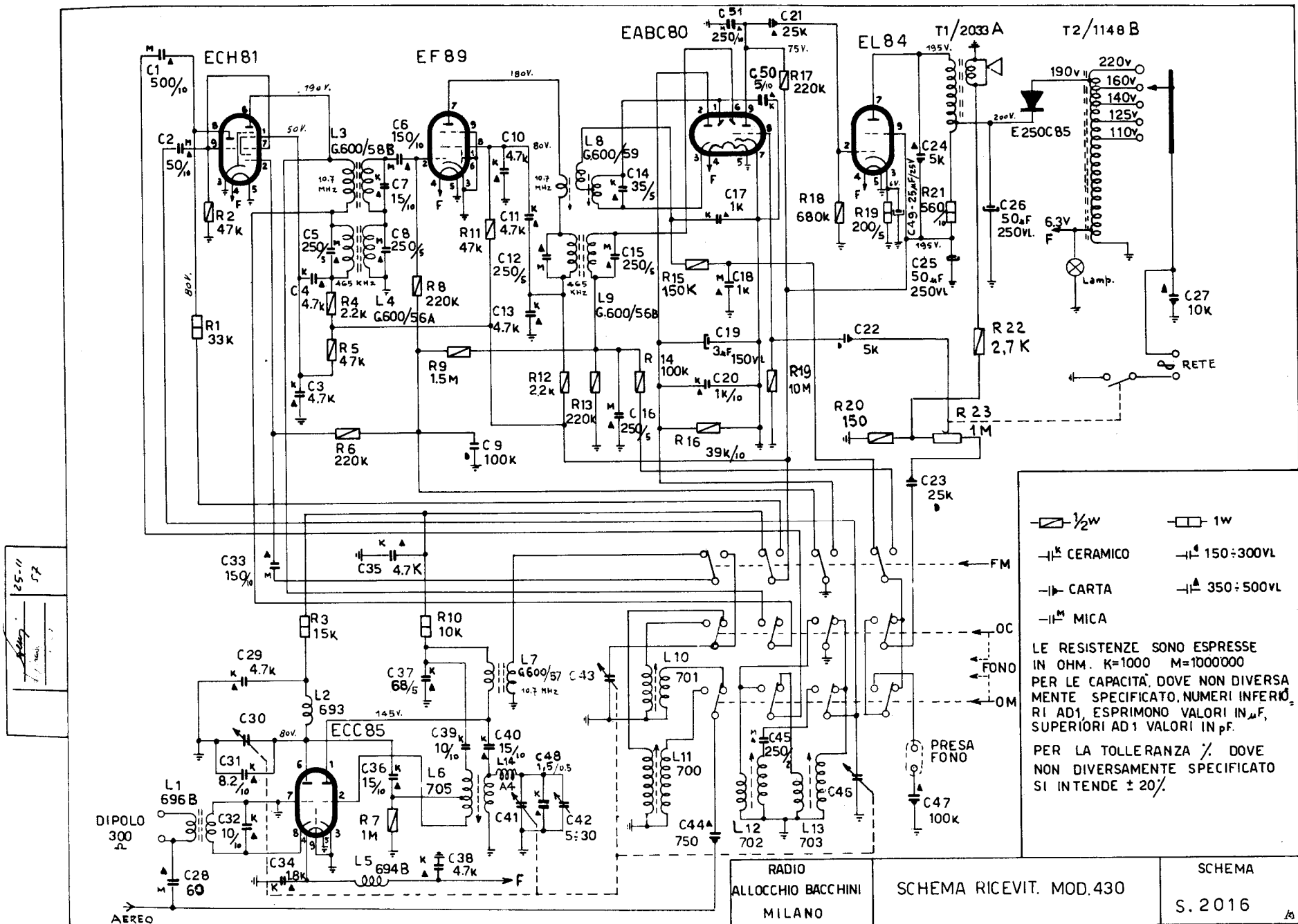
RADIO ALLOCCIO BACCHINI - Mod. 430. Apparecchio AM/FM con una gamma onde medie, una gamma onde corte e una gamma onde ultracorte. Commutatore in posizione FM. Medie frequenze a 465 kc/s e a 10,7 Mc/s. Potenza d'uscita 2,5 watt. Consumo 45 watt. (V. retro tabella tensioni e resistenze).
